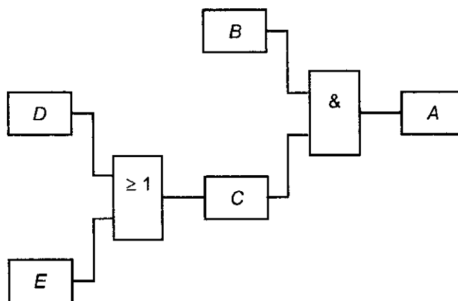
Рисунок 1 — Пример дерева неисправностей
