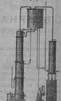
Винокуренный аппаратъ.
