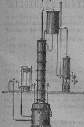
Спирто-ректификаціонный аппаратъ.
