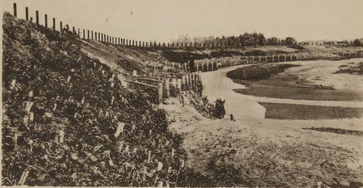
Укрѣплєніе берега р. Бездны у д. Халанѣвки Гусихинской вол. Спасскаго у. Казанской губ.
