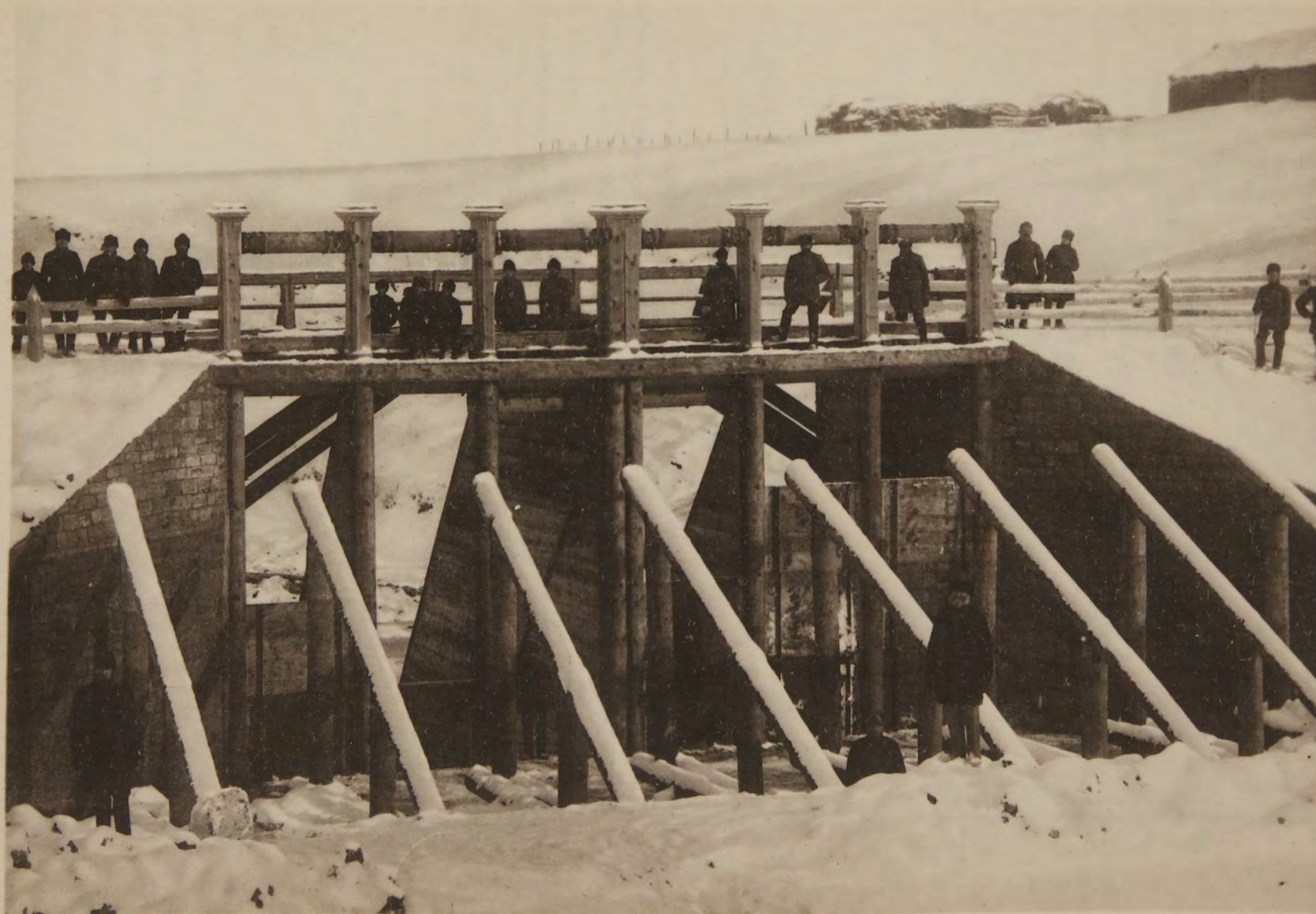
Водоспускъ на запрудѣ въ с. Клопихѣ Карнѣевской вол. Николаевского у. Самарской губ.
