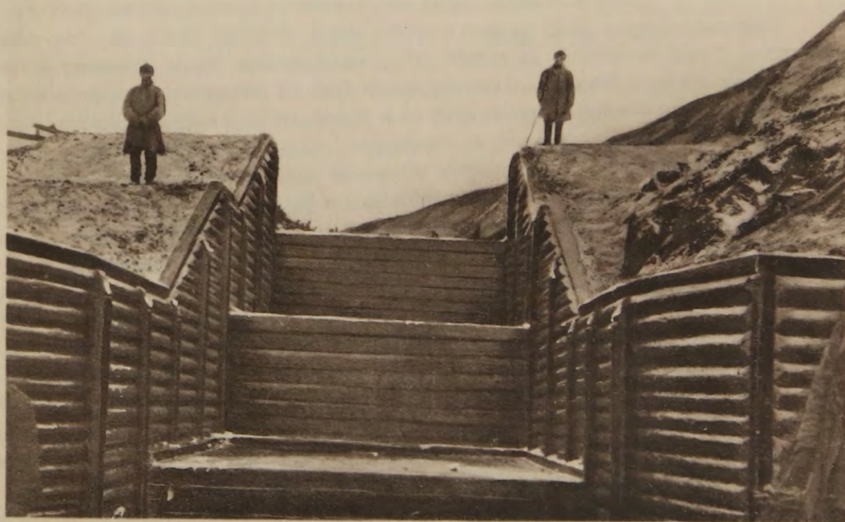
Водосливъ „Молокановской“ плотины села Брыковки Никольской вол. Николаевского у. Самарской губ.
