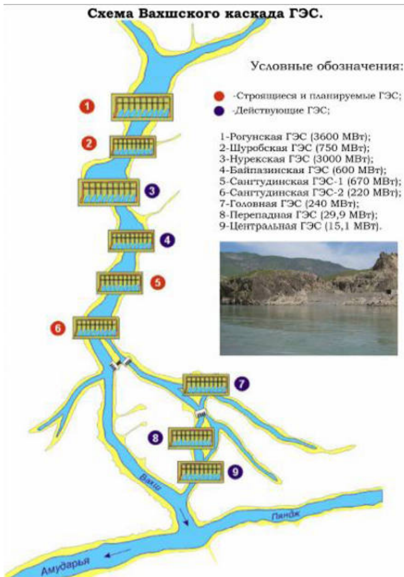
Рис. 5. Схема комплексного использования Вахшского каскада
