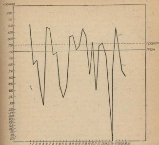
Диаграмма 1. Суточная выплавка чугуна из домновой печи № 2 Кузнечного завода в августе 1933 г.
