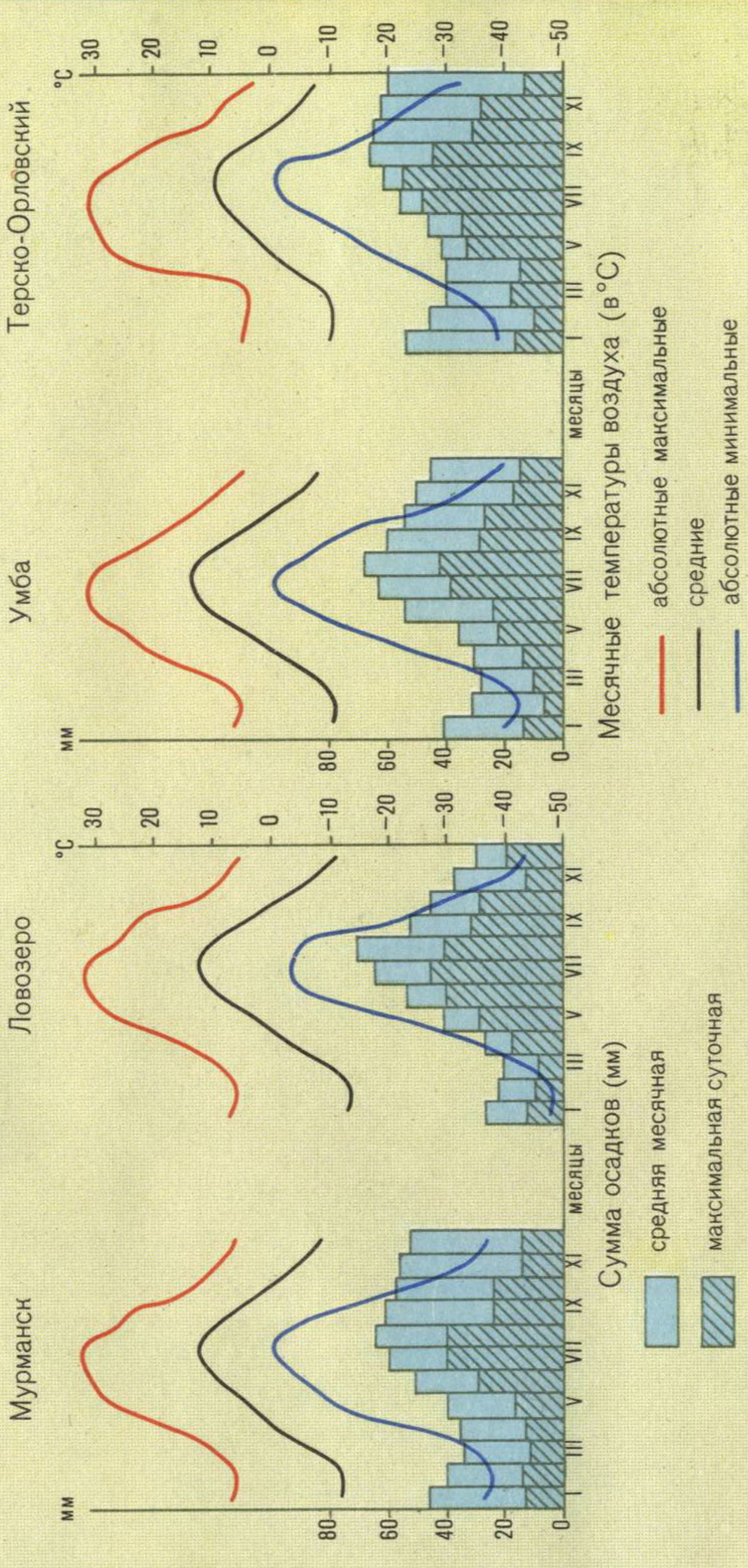
ГОДОВОЙ ХОД ОСАДКОВ И ТЕМПЕРАТУРЫ ВОЗДУХА
