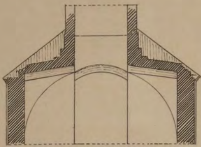
Разрез по линии АВ. Черт. 2 я .
