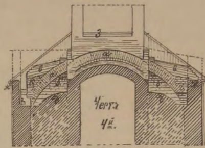
Фасадъ свода въ поперечной стѣнѣ В.
