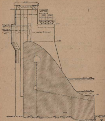
№ 5. Поперечный разрез по водонепроницаемой части плотины
