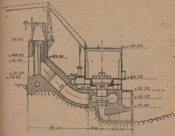
№ 6. Поперечный разрез гидростанции по оси большой турбины
